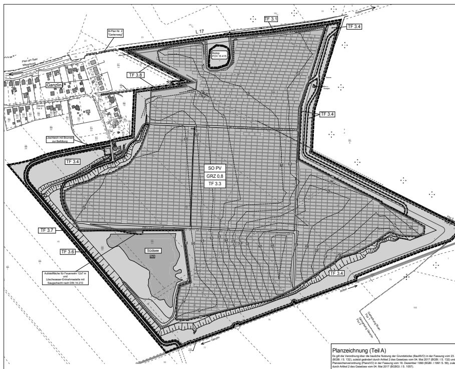
Satzung der Gemeinde Ganzlin über den vorhabenbezogenen B-Plan Nr. 14 „Photovoltaikanlage Kieswerk Ganzlin“ der Gemeinde Ganzlin · M 1:2.500 Gemarkung Ganzlin, Flur 2 und 3 · Plangebietsgröße: 68,7 ha
