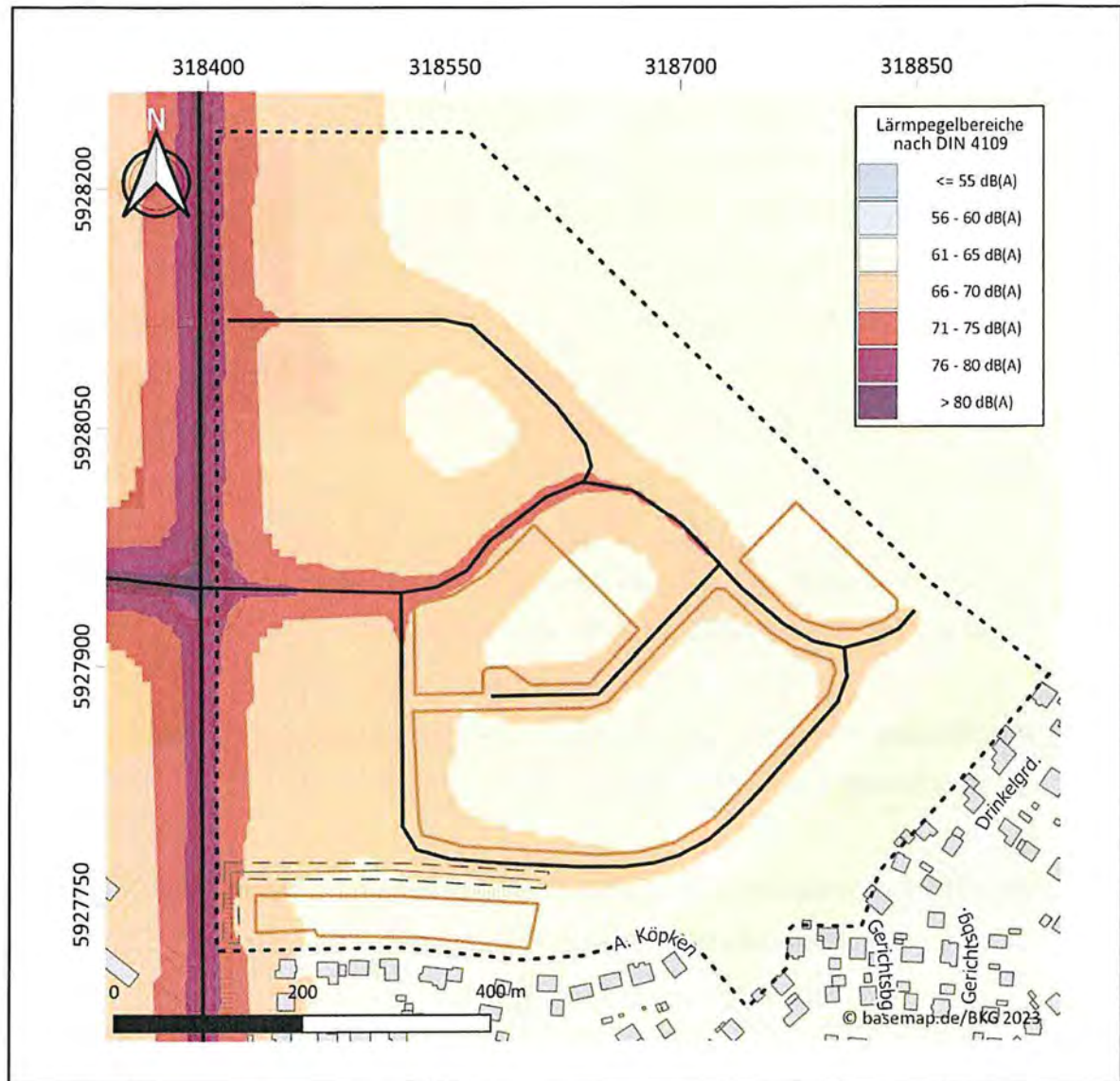
Abbildung 20: Lärmpegelbereiche für Mischgebiete nach DIN 4109-1 (Höhe 5 m)
