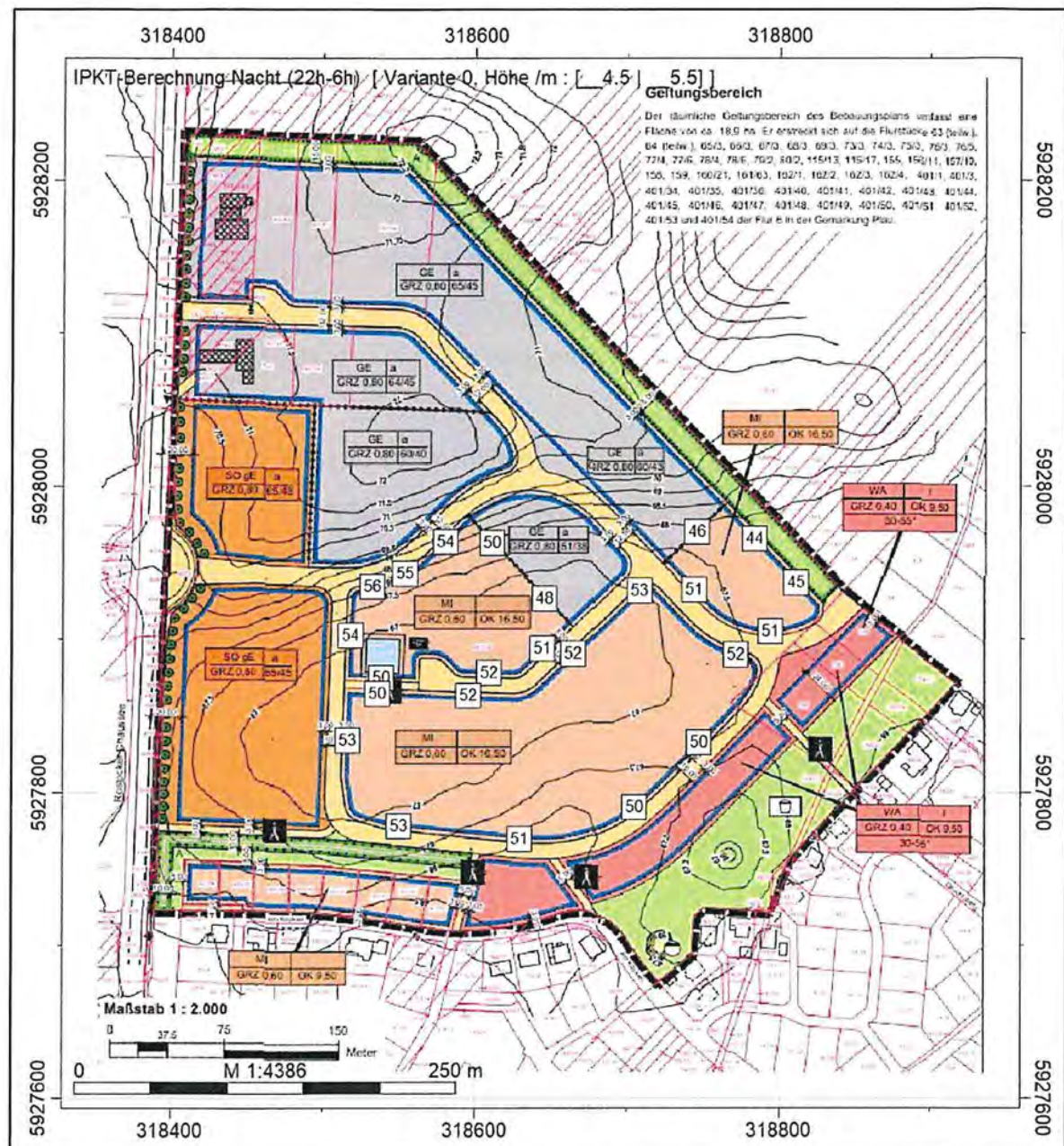
Abbildung 16: Beurteilungspegel für die Beurteilungszeit Nacht (22.00 bis 6.00 Uhr), 1. Obergeschoss (Höhe 5 m)
