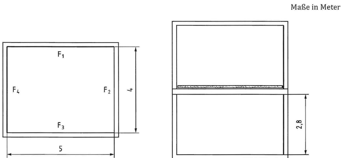
Bild D.3 — Grundriss (links) und Schnitt (rechts) zweier übereinanderliegender Räume im Holzbau (Prinzipskizze)
